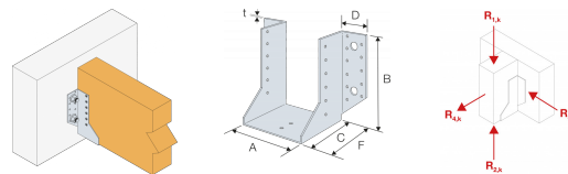
Valeurs Caractéristiques - Bois sur béton ou acier
